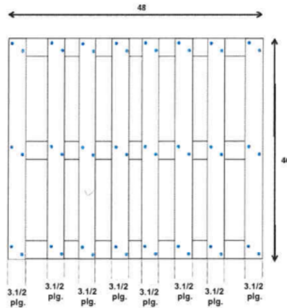
VISTA SUPERIOR
